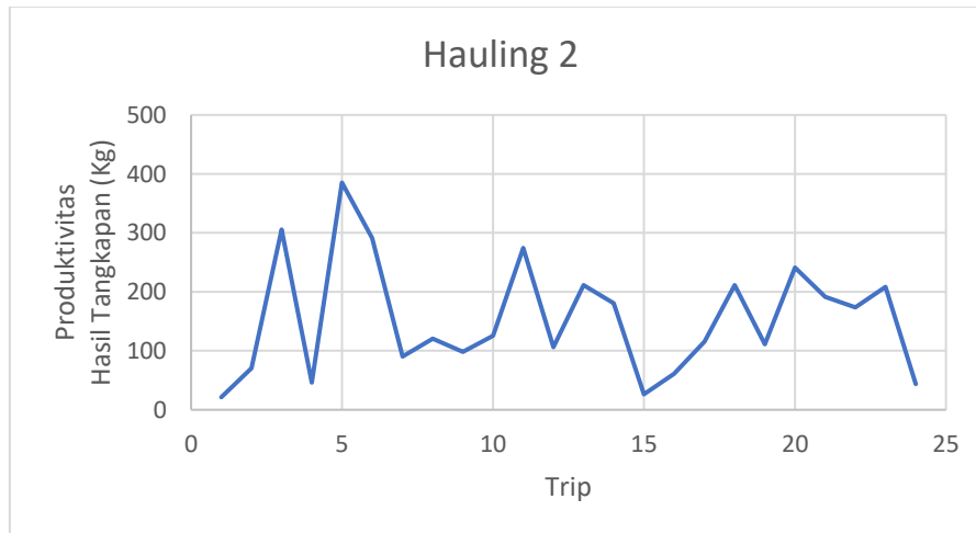
Gambar 2. Grafik nilai produktivitas tertinggi pada hauling kedua
