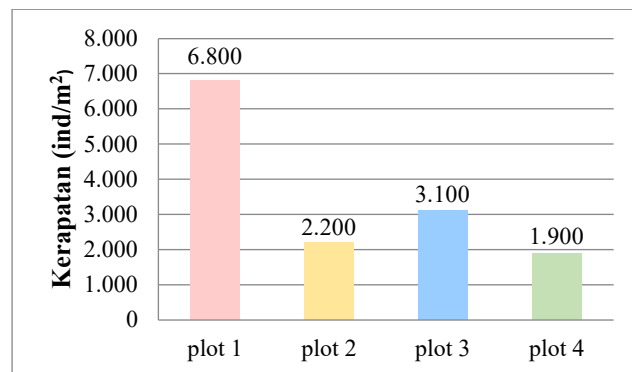
Gambar 2. Kerapatan Mangrove
