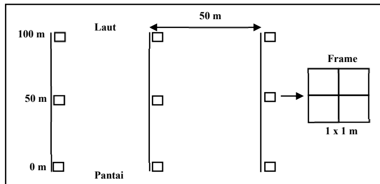
Gambar 2. Skema Transek Kuadran
