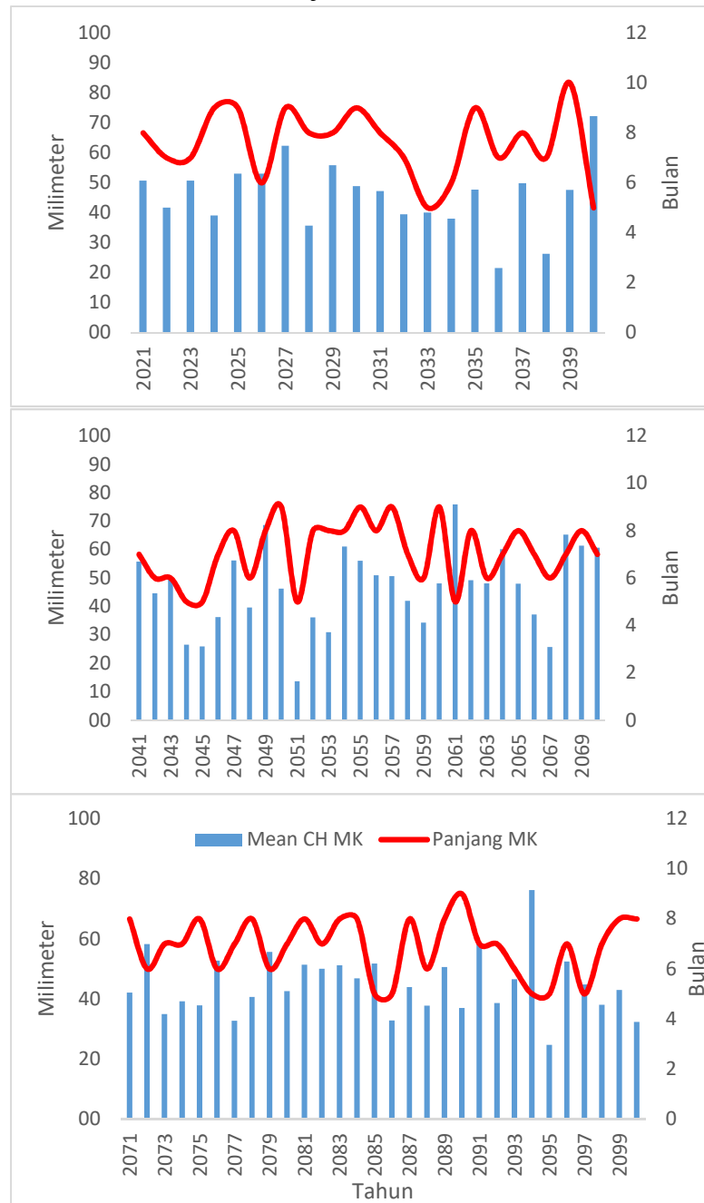
Gambar 3. Rerata curah hujan dan panjang musim kemarau di Jeneponto bagian barat periode 2021 – 2100
