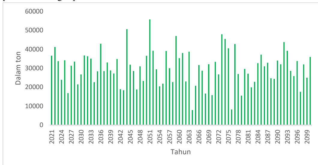
Gambar 5. Perkiraan produksi garam tahun 2021-2100
