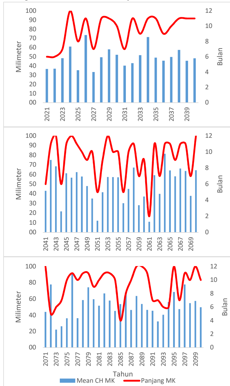
Gambar 4. Rerata curah hujan dan panjang musim kemarau di Jeneponto bagian timur periode 2021 – 2100
