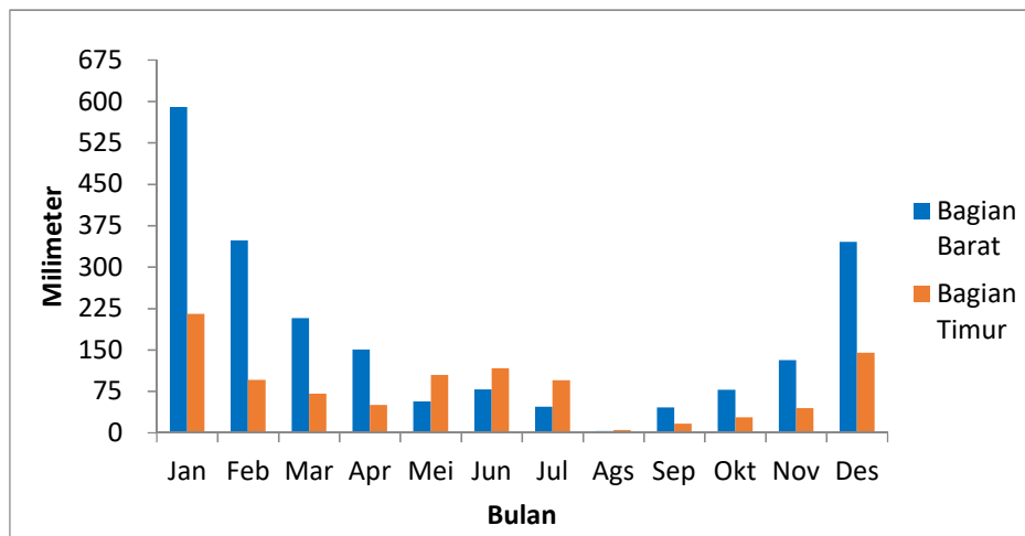
Gambar 2. Curah hujan di Jeneponto tahun 2009-2018
