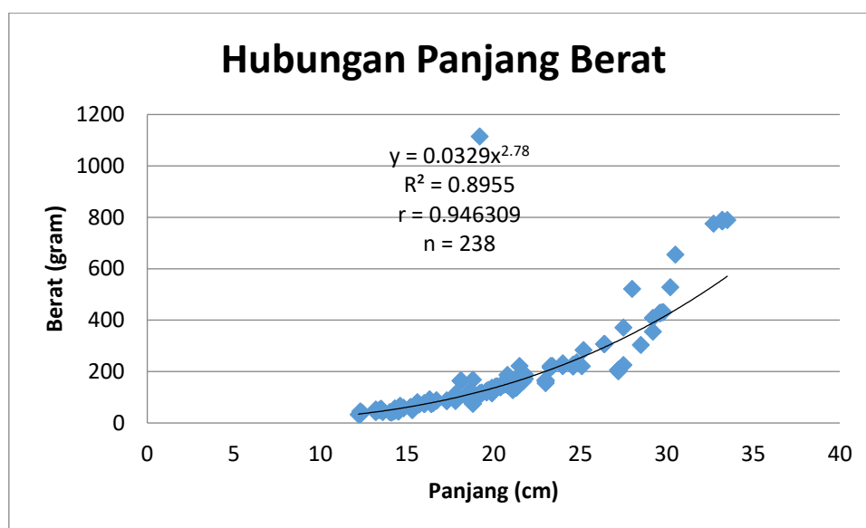
Gambar 4. Hubungan Panjang Bobot Ikan
