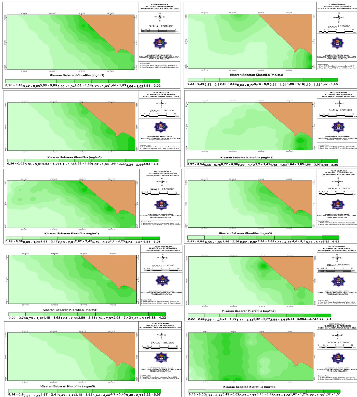
Gambar 3. Peta sebaran klorofil-a dari bulan Januari - Oktober 2022 di perairan Aceh Barat. Figure 3. Chlorophyll-a distribution map from January - October 2022 in West Aceh waters.
