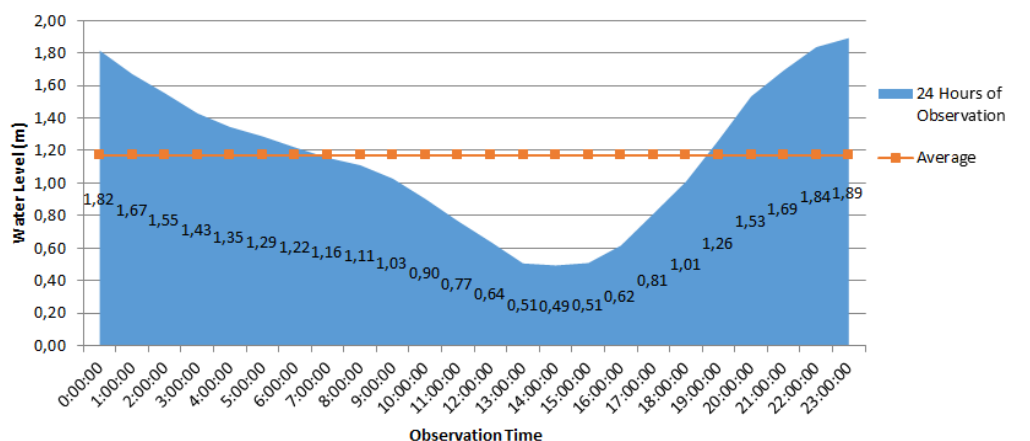
Gambar 2. Pola Pasang Surut di Kawasan Mangrove Lantebung
